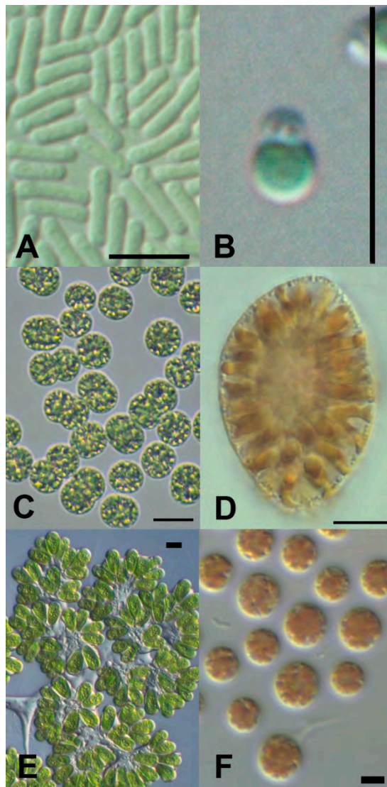
A. Thermosynechococcus (NIES-2133), B. Cyanidioschyzon (NIES-1332), C. Microcystis (NIES-44), D. Chattonella (NIES-3), E. Botryococcus (NIES-836), F. Porphyridium (NIES-1035). Scale bar = 10 \mu\text{m} .
